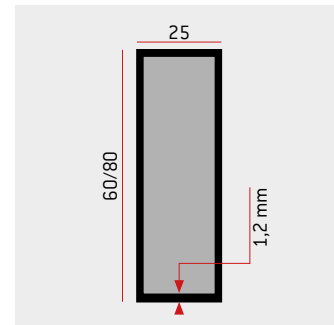
Profile o przekroju 1,2 mm Sides with 1,2 mm section
